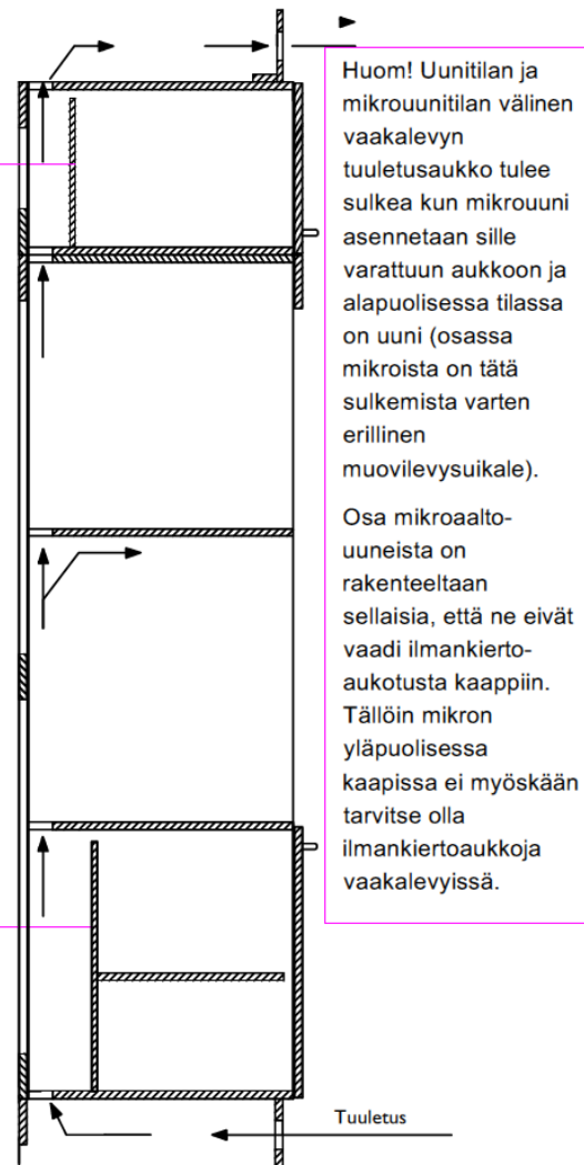
Leikkaus A-A
